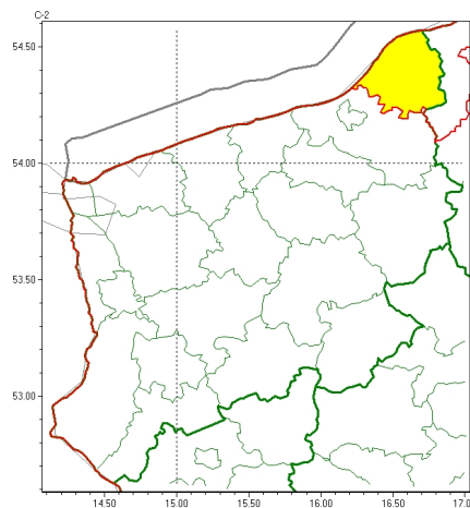
Silny wiatr 2024-04-05 11:42
