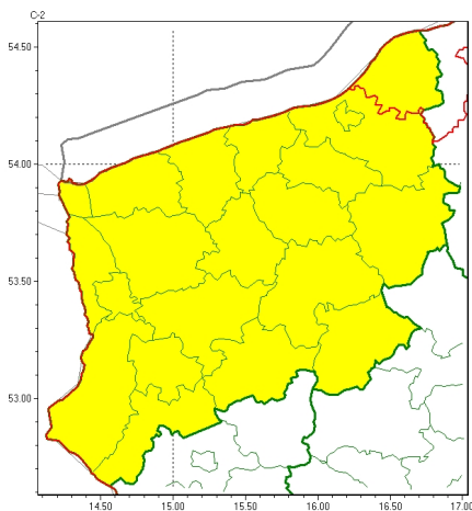
Burze 2024-04-05 11:42
