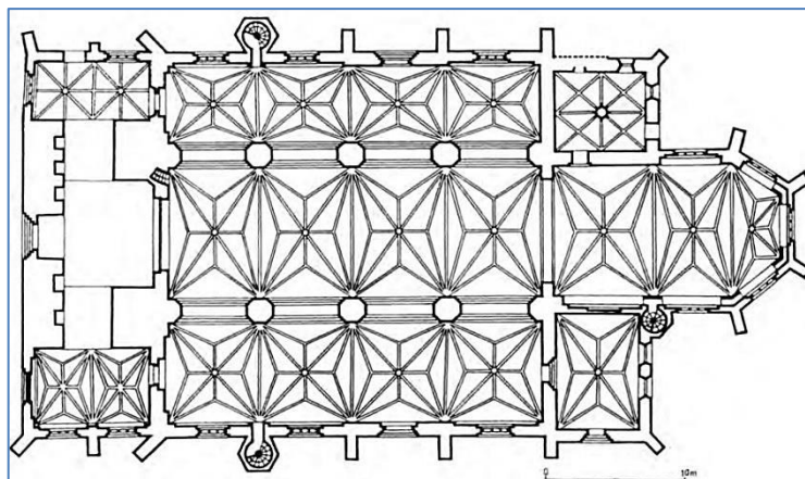
Rzut planu kościoła pw. (.) Matki Boskiej Częstochowskiej
